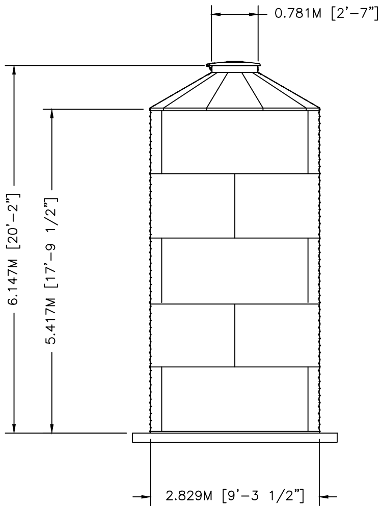
ELEVATION
