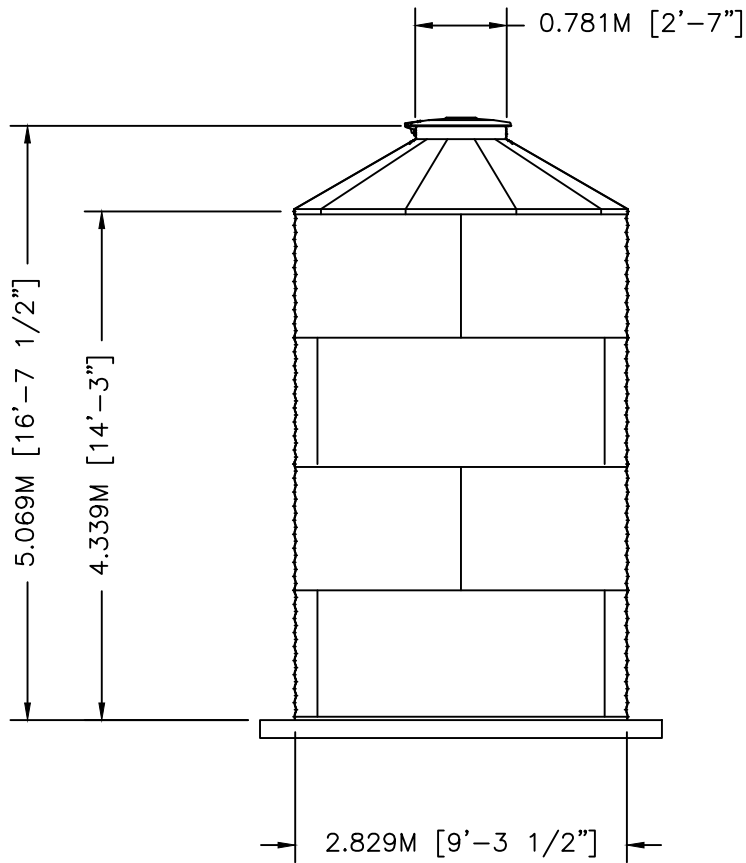
ELEVATION
