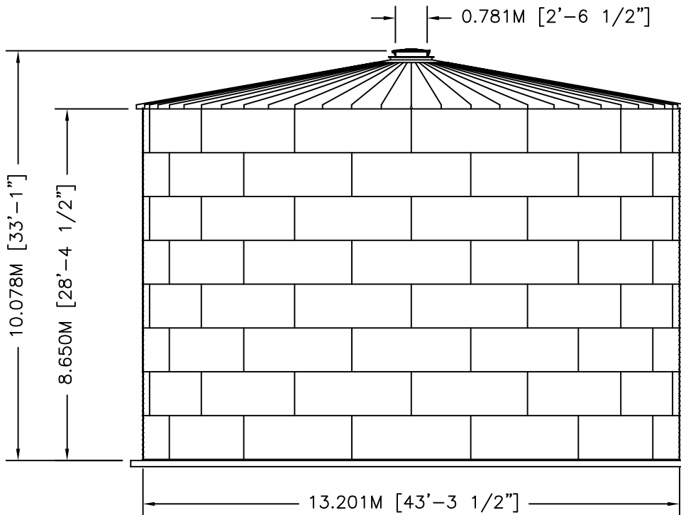
ELEVATION
