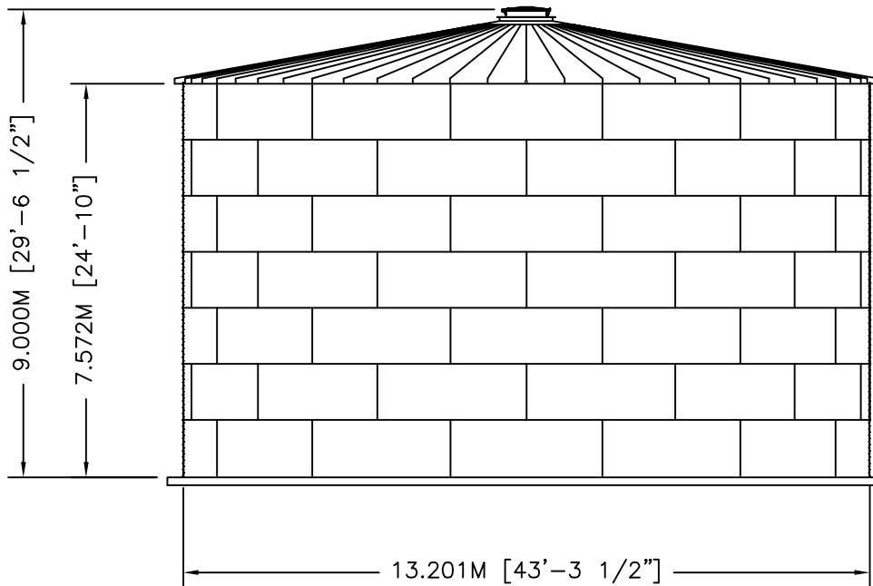
ELEVATION
