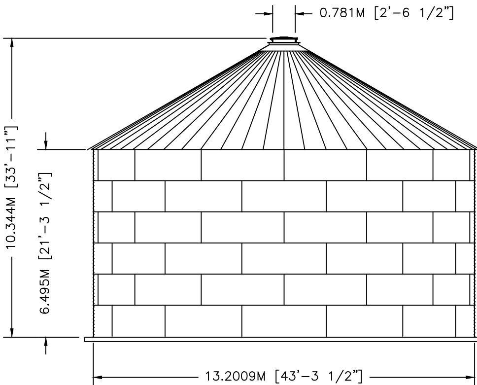
ELEVATION
