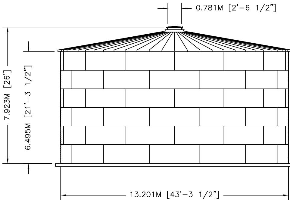
ELEVATION
