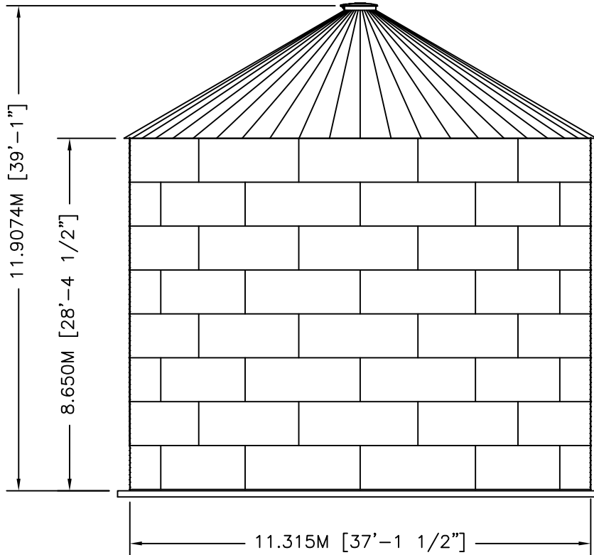
ELEVATION
