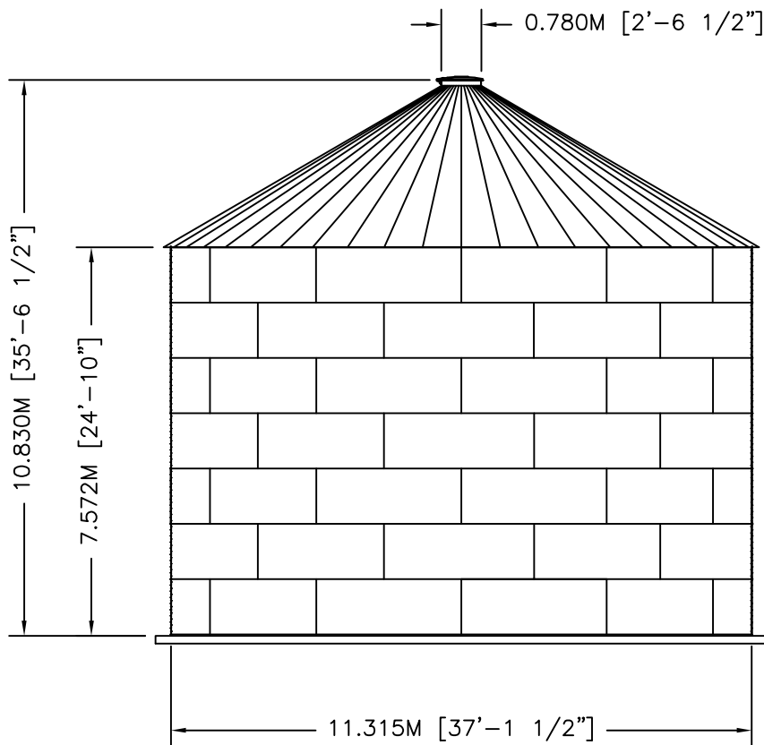
ELEVATION
