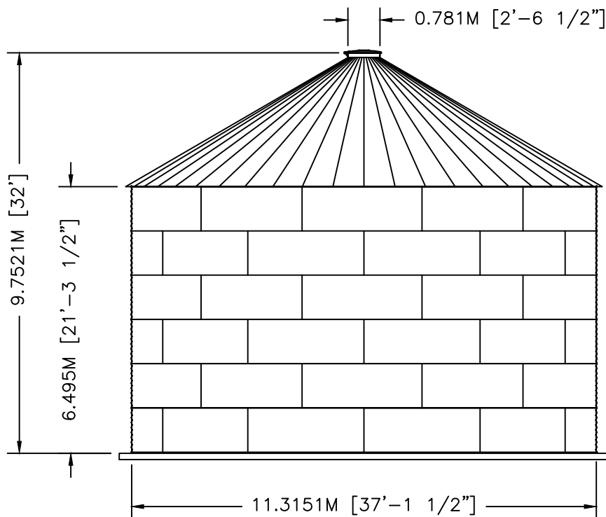
ELEVATION
