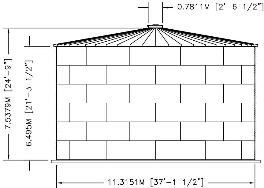
ELEVATION
