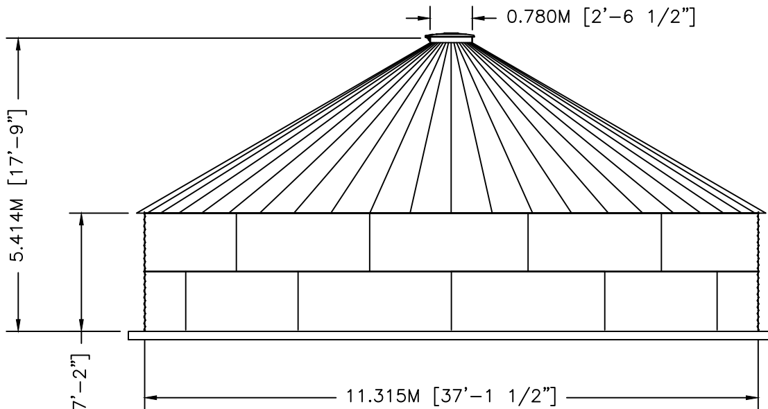
ELEVATION
