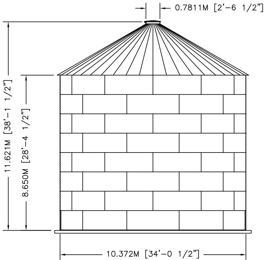
ELEVATION
