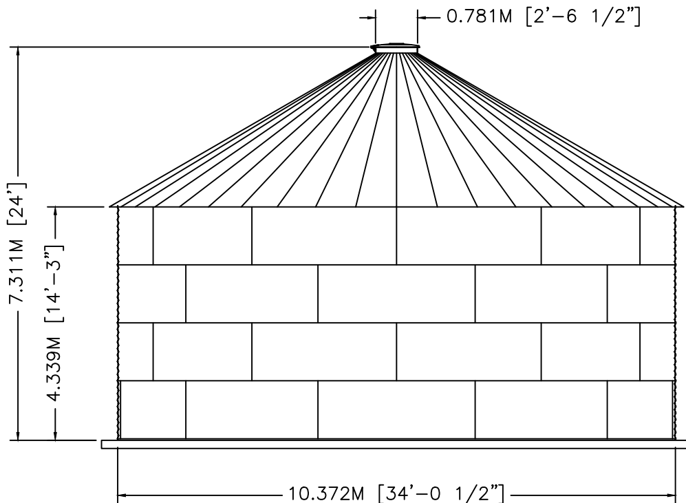
ELEVATION
