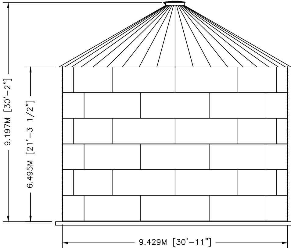
ELEVATION
