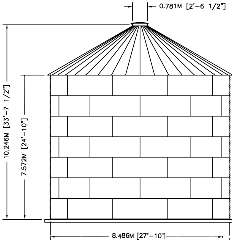
ELEVATION
