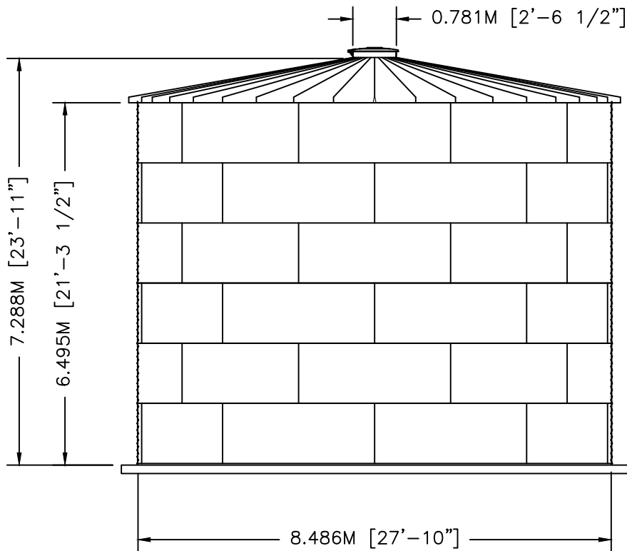
ELEVATION
