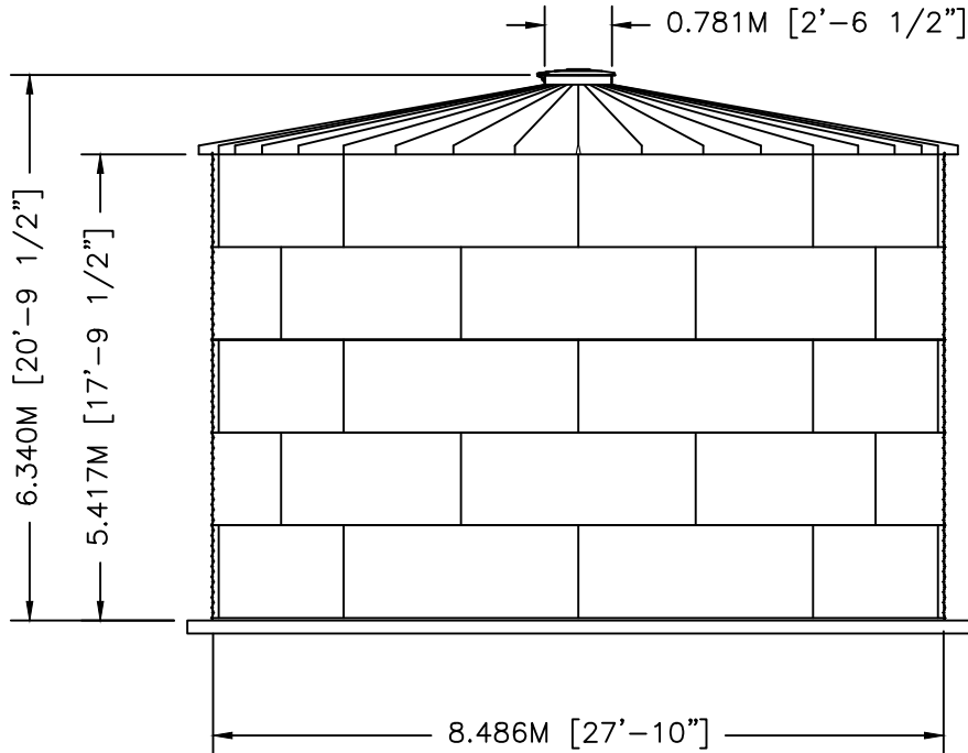
ELEVATION
