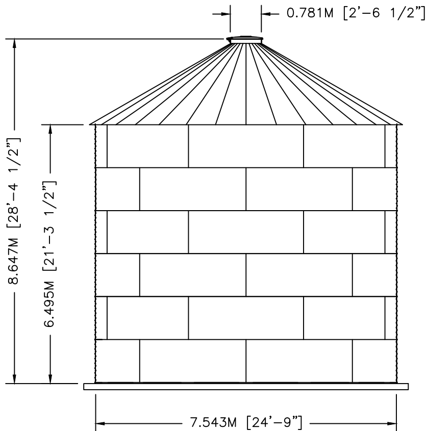
ELEVATION
