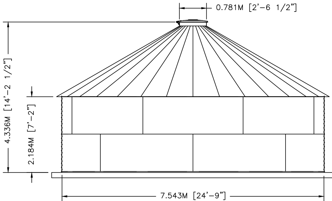
ELEVATION
