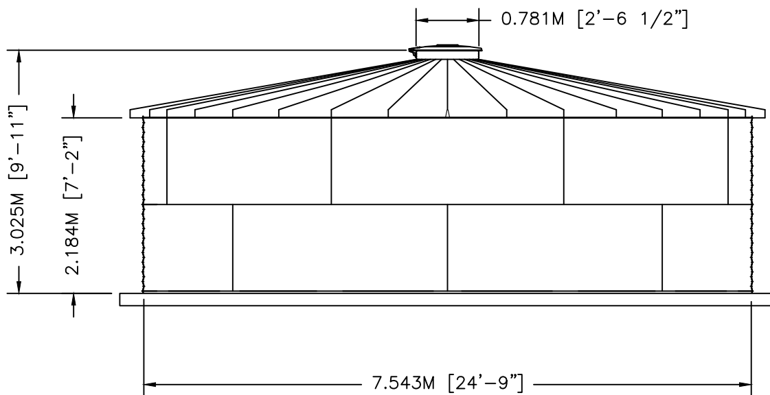
ELEVATION
