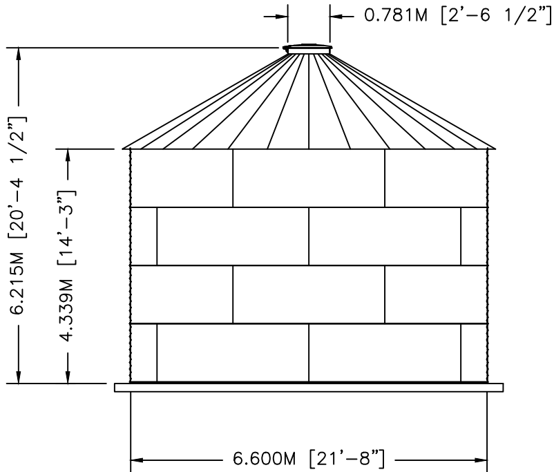
ELEVATION
