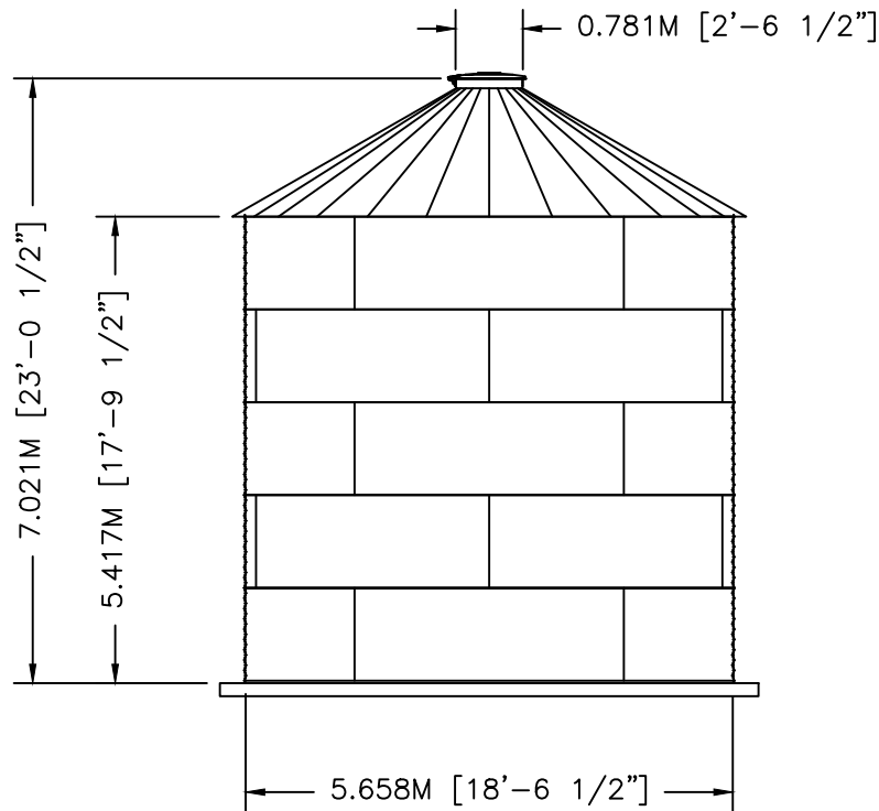
ELEVATION
