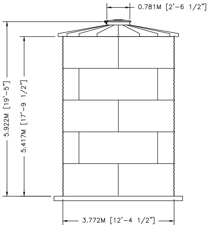
ELEVATION
